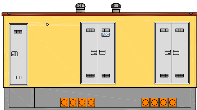
PROSPETTO FRONTALE
